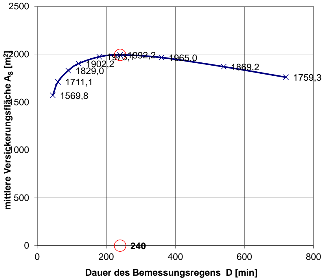
Muldenversickerung
